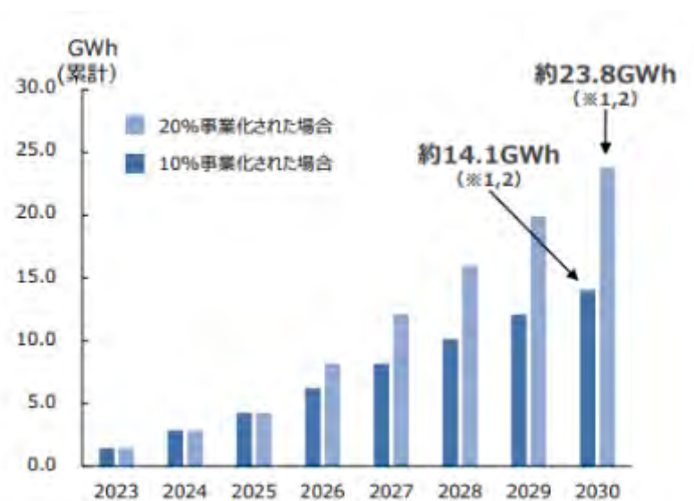
図 1 - 10 系統用蓄電池の導入見通し
